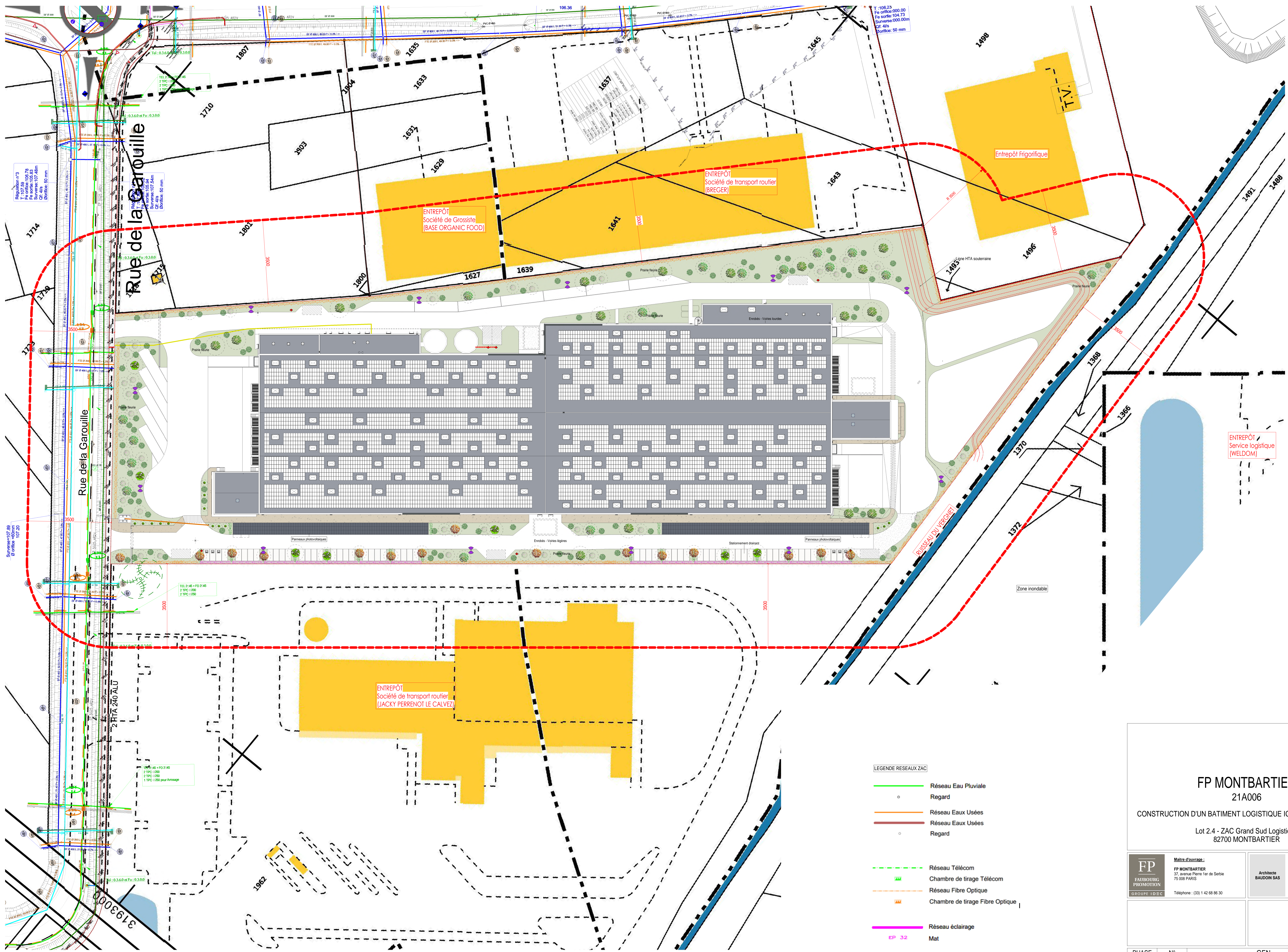
Plan de masse Ech: 1:500
